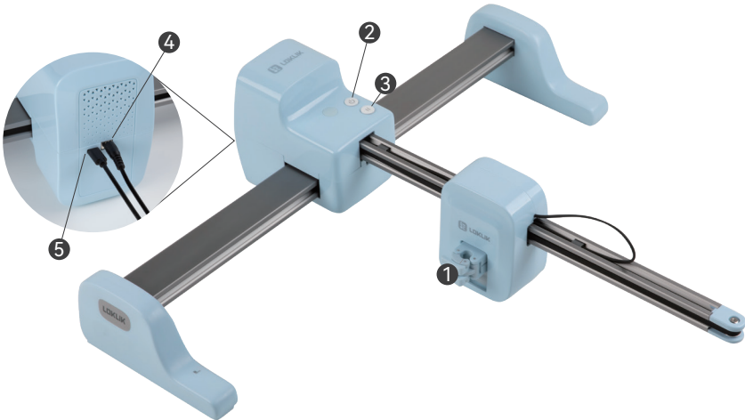
1.笔座 2.电源键 3.暂停键 4.电源接口 5.Type-C数据接口
